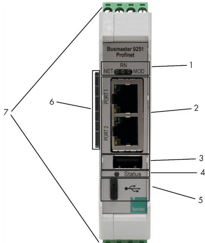
Abbildung: 3 Frontansicht Feldbus-Controller Typ 9251.
